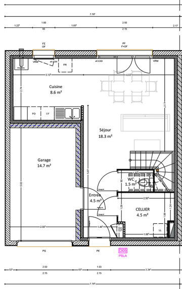
PLAN RDC
